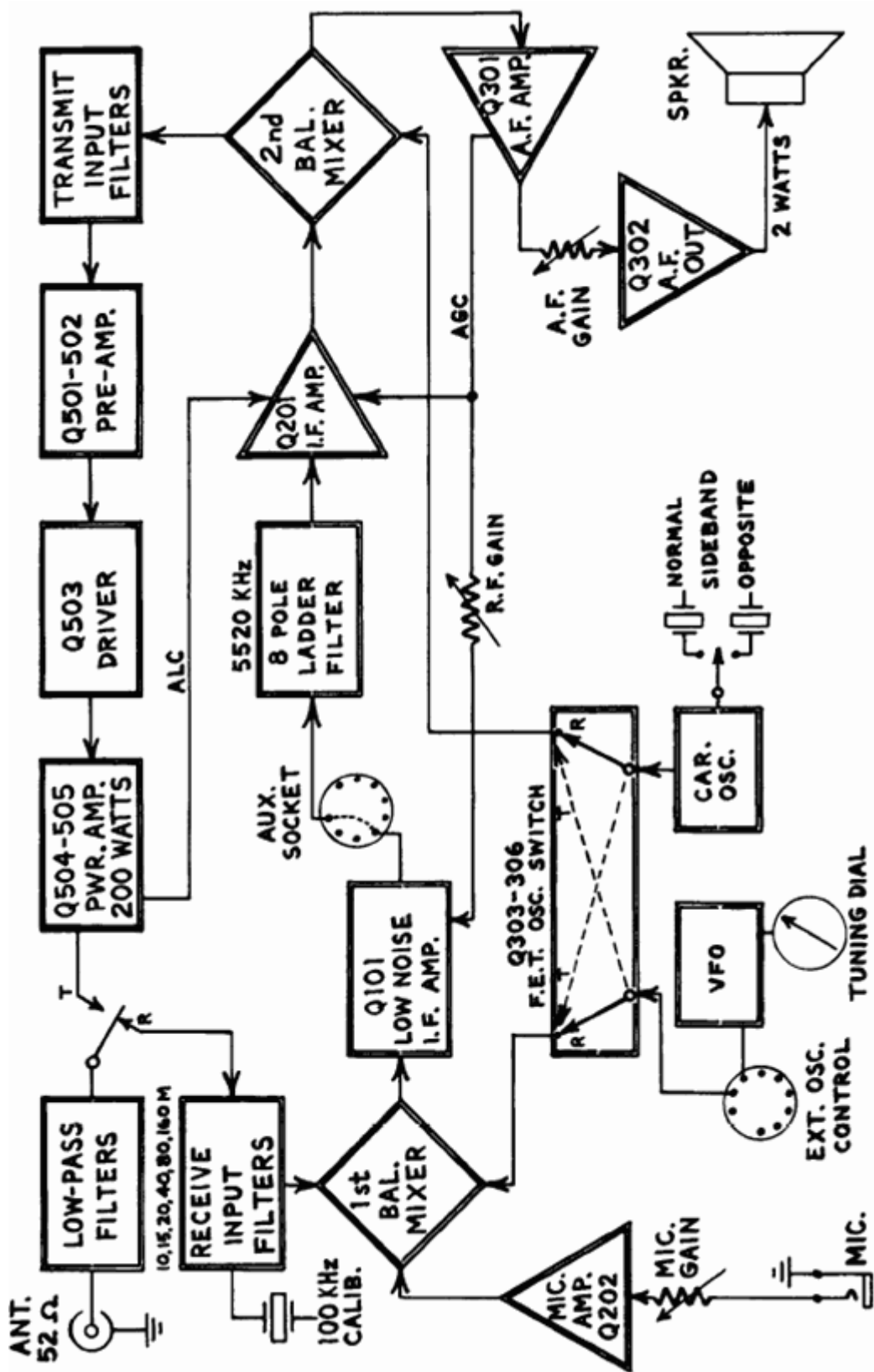
Rysunek 4-2. Schemat blokowy ATLAS 210x/215x
