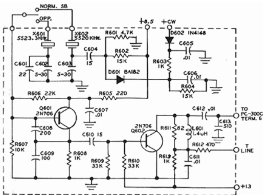
Rysunek 4-9. PC-600 Schemat elektryczny oscylatora Colpittsa
