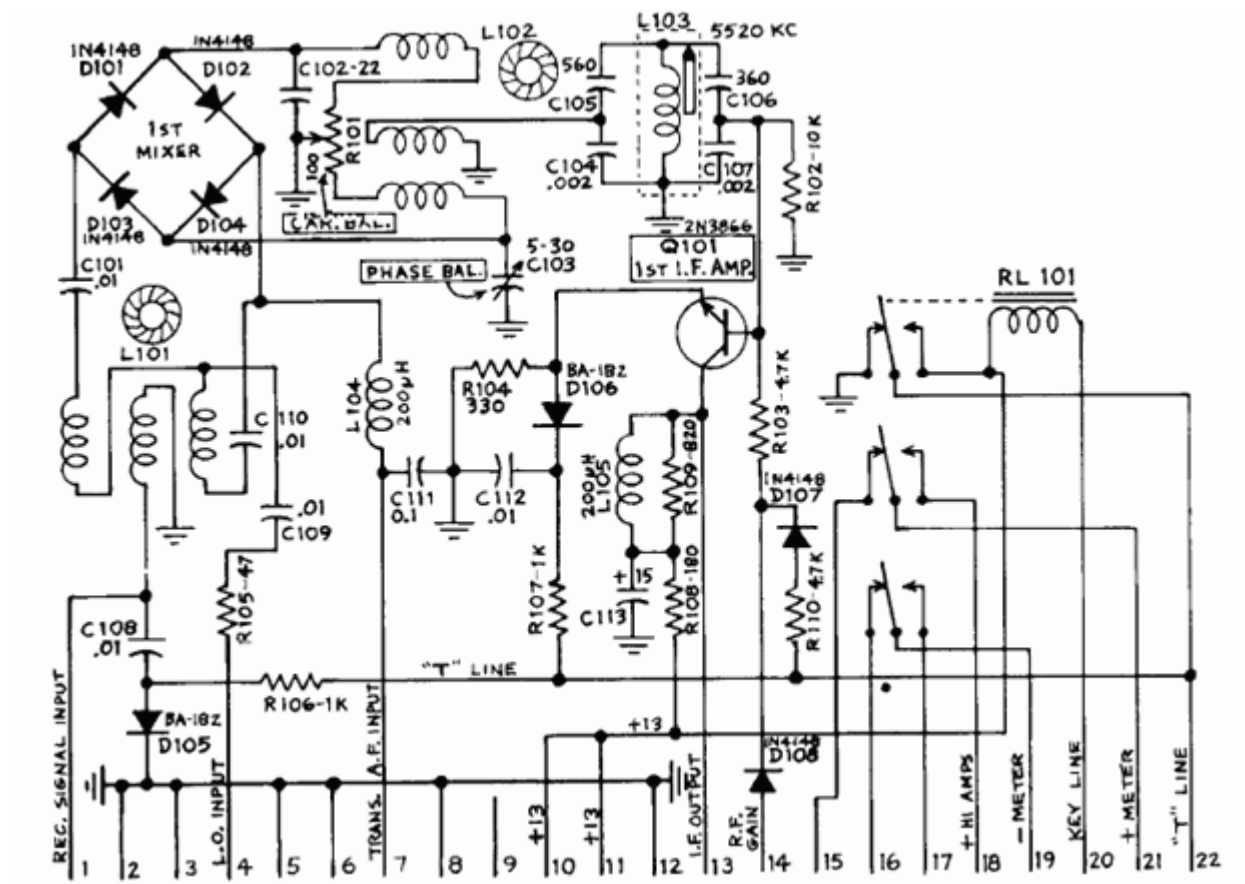
Rysunek 4-4. PC-100A Schemat elektryczny
