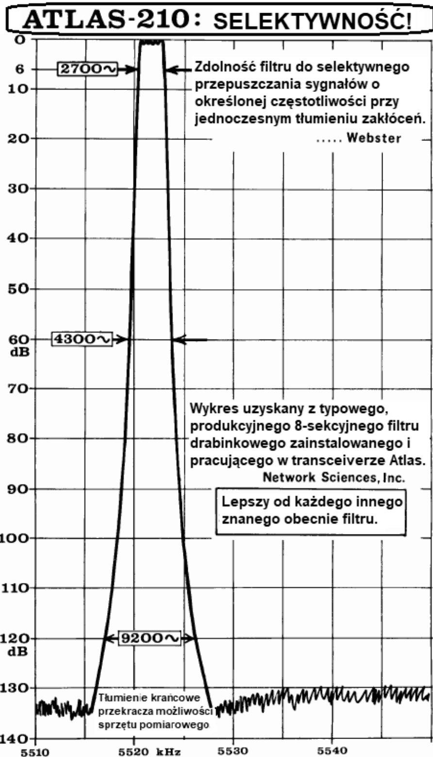
Rysunek 4-3. Charakterystyka selektywności filtru drabinkowego kwarcowego
