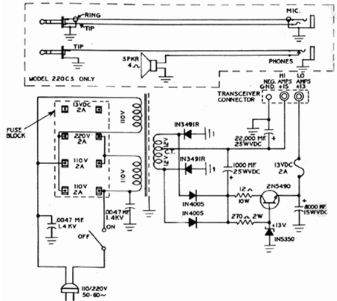
Rysunek 2-7. Schemat modelu 220-CS/200-PS
