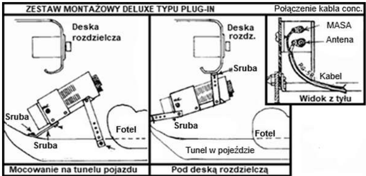
Rysunek 2-3. Instalacja zestawu montażowego typu plug-in Deluxe
