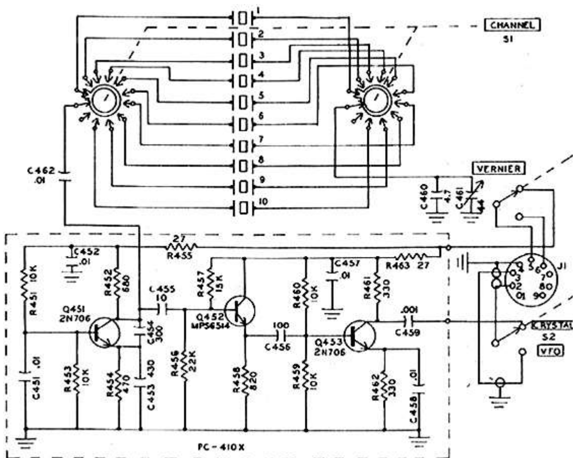
Rysunek 5-3 Schemat Oscylatora Kwarcowego Model 10x
