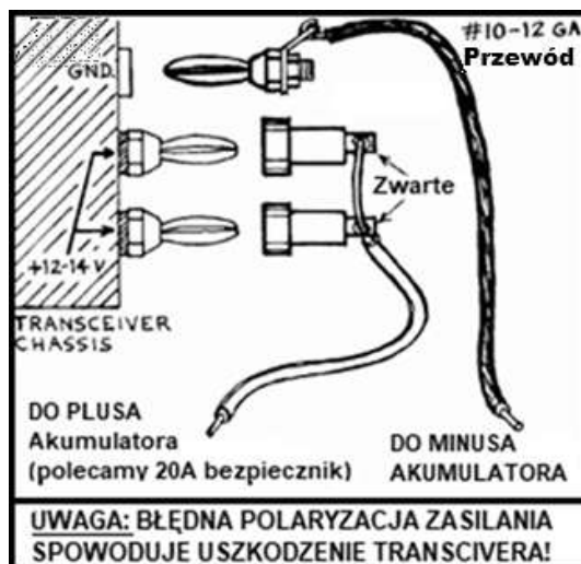
Rysunek 2-5. Połączenia zasilania stałego
